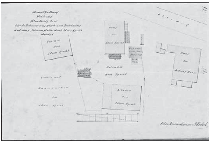
Lageplan Backhaus Bauernhof Specht
